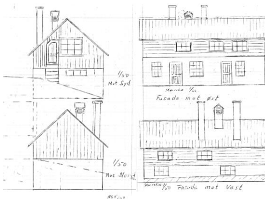
Byggetegninger til renserisøknad i 1947
